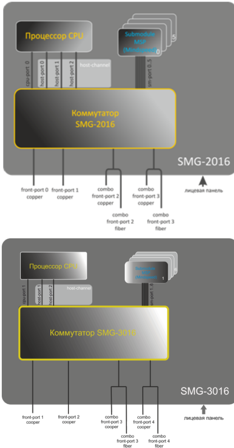
Рисунок 49 – Структура коммутатора
