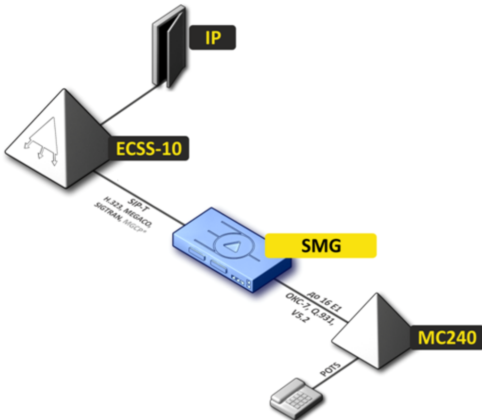
Рисунок 2 – Сопряжение сигнализаций и медиапоточков TDM- и VoIP-сетей
